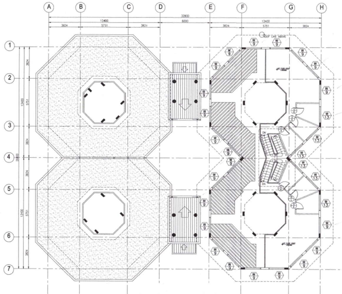
1 LOFT REFERENCE PLAN A-3 SCALE 1:150 M.
